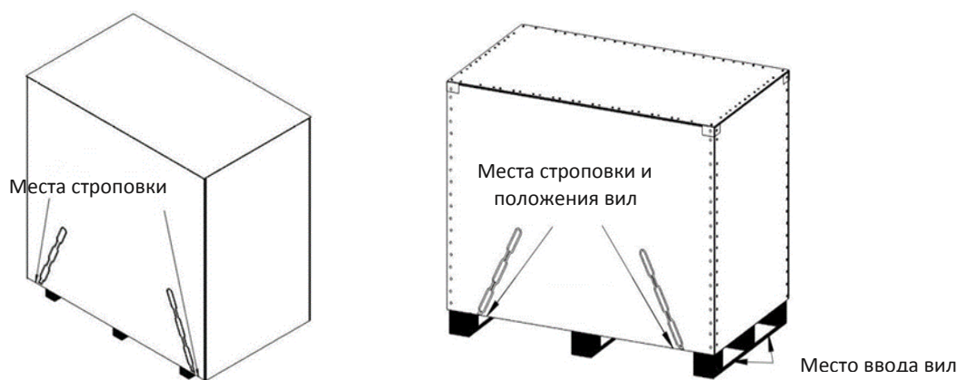
Рис. 2.5 - Строповка (паллеты с выступом - слева, паллеты без выступа - справа)
