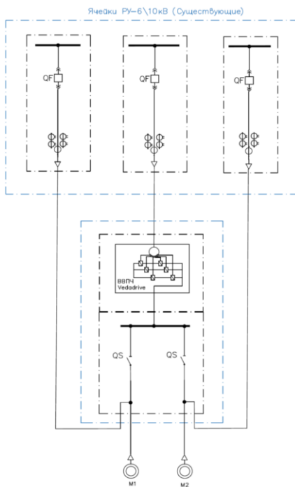
Рис. 6.5 - Схема переключения рабочий-резервный ручной
