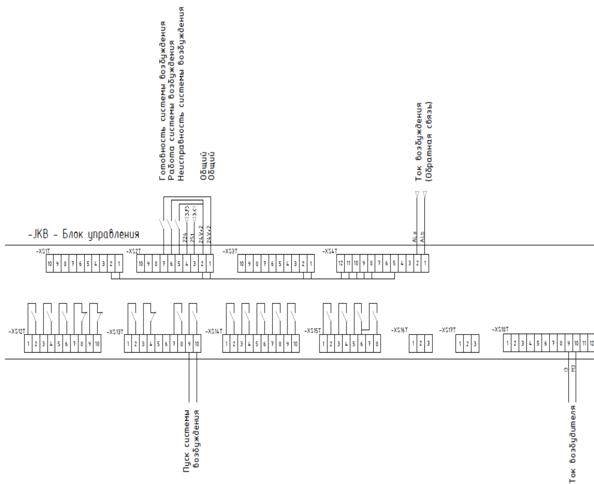
Рис. 8.6 - Схема подключения возбудителя к ПЧ
