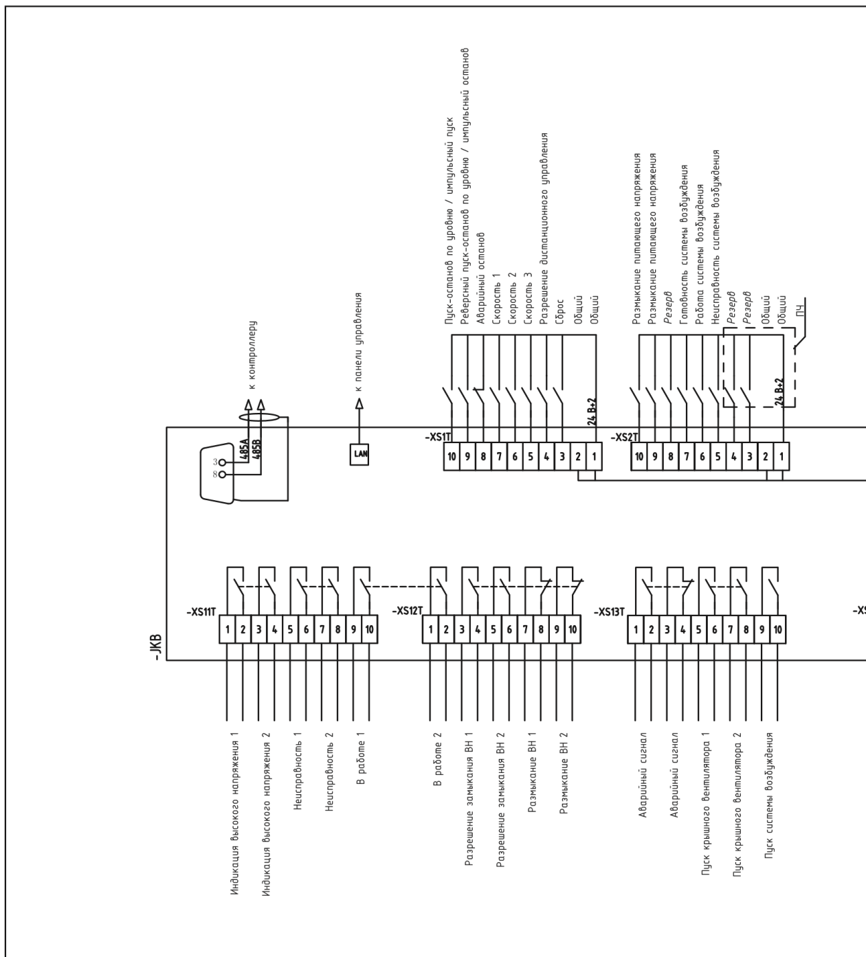
Рис. 3.3 - Электрическая схема подключения цепей управления
